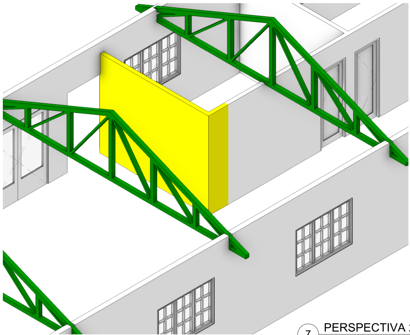
7 PERSPECTIVA 2 Escala: 1:50
