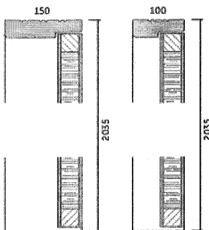
MARCO DE MADERA
