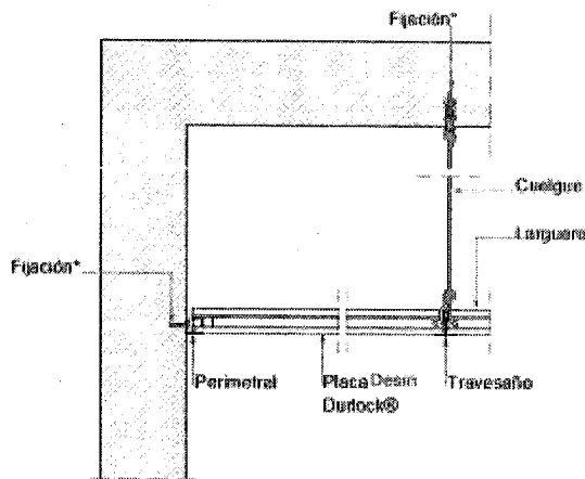
Encuentro con Pared Durlock.
