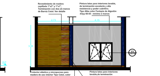
CORTE D-D
