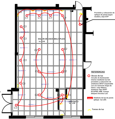
PLANTA - INSTALACION ELECTRICA
