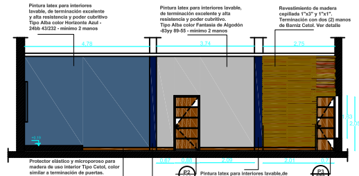
CORTE C-C
