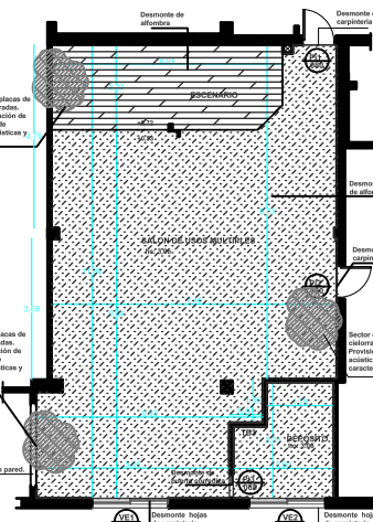
SUM- Salón de Usos Múltiples PLANTA EXISTENTE Esc:1/75
