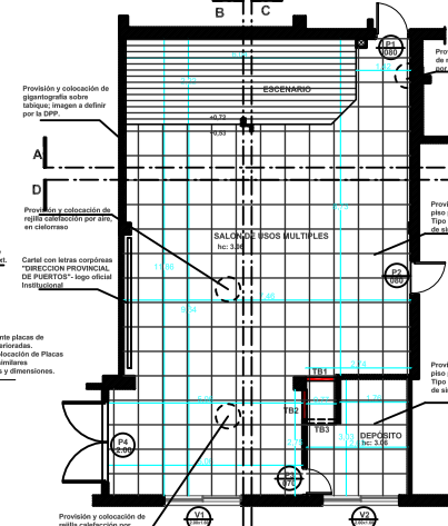
SUM- Salón de Usos Múltiples PLANTA - REMODELACION Esc:1/75
