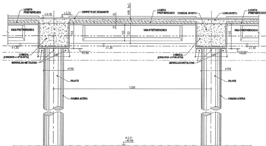
CORTE LONGITUDINAL
