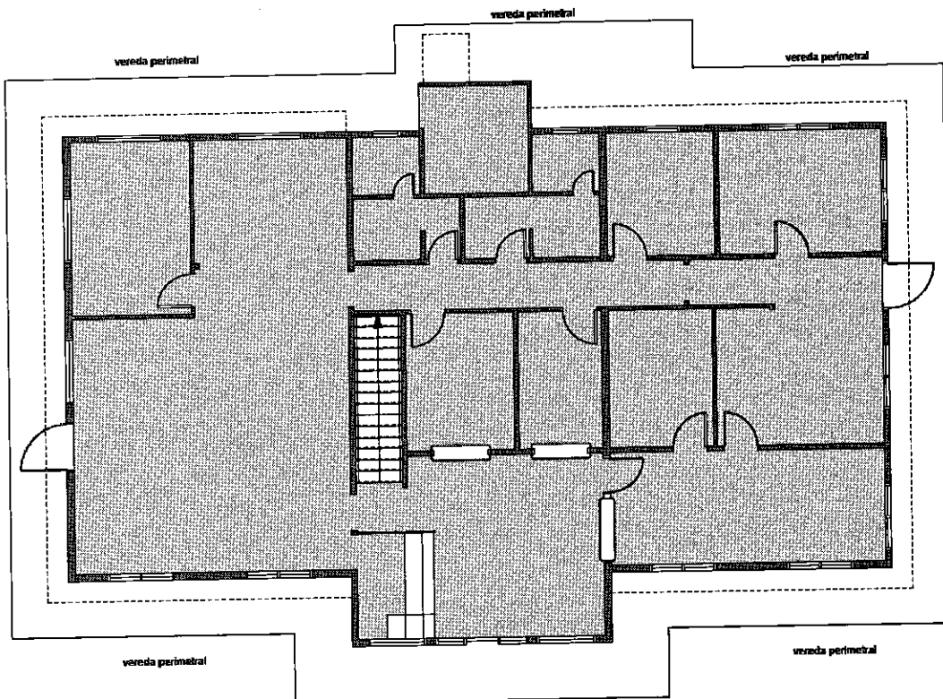
PLANTA BAJA SUP. 198.73m 2
