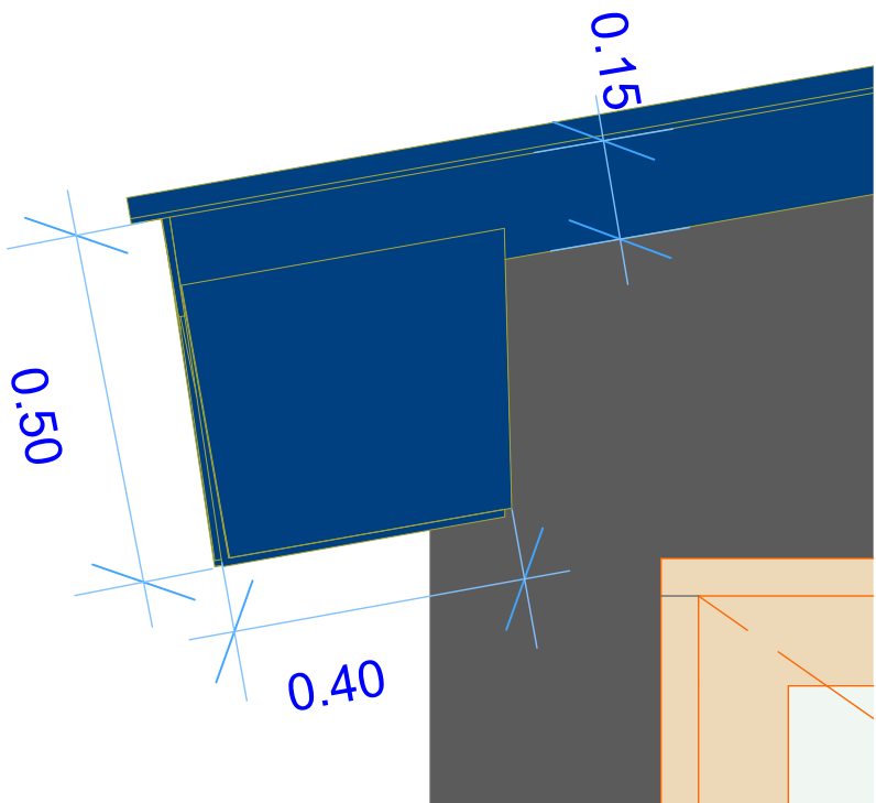
DETALLE ALERO CUBIERTA TALLER
